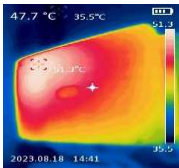
inverter No3 อุณหภูมิ 51.3 °C
