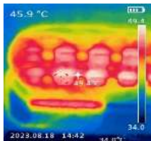
ภายในตู้ combination box อุณหภูมิ 49.4 °C
