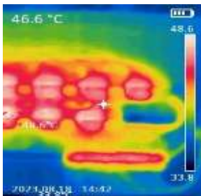
ภายในตู้ combination box อุณหภูมิ 48.6 °C
